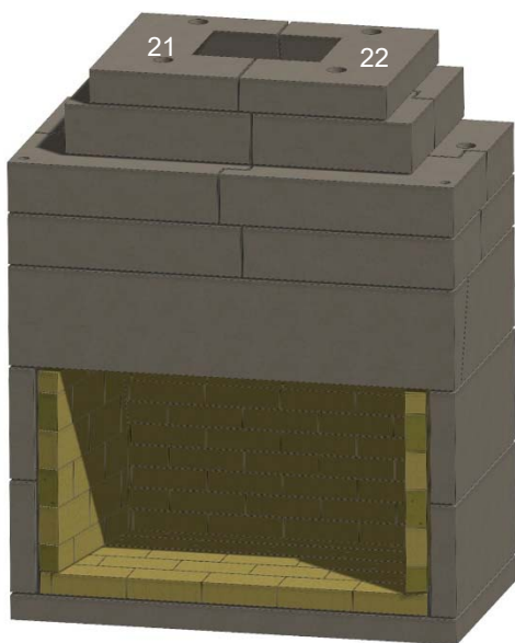
Figure 16. Capuchon de gorge
