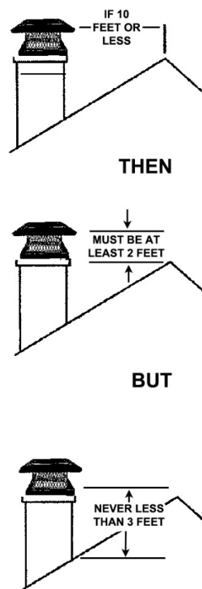
Figure 25. Hauteur de la cheminée
