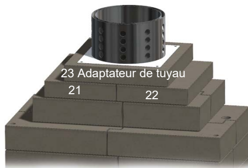
Figure 18. Cheminée en tube métallique
