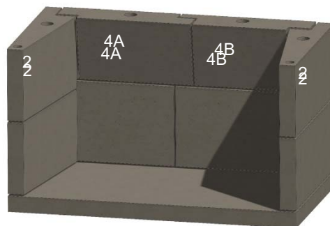
Figure 6. Plaques dorsales et parois latérales du milieu
