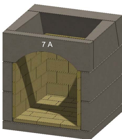
Figura 18. Dintel frontal
