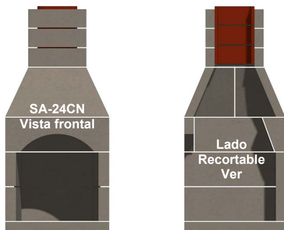
Figura 1. Montaje de la chimenea SA-24CN & Vista en corte
