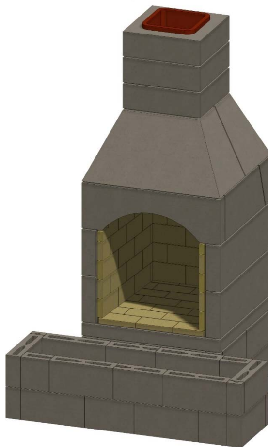
Figura 22. Base de la chimenea
