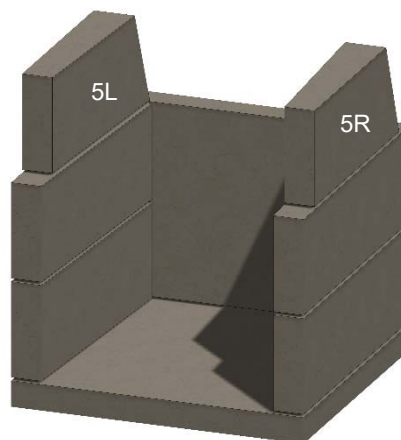
Figura 13. Paredes laterales superiores
