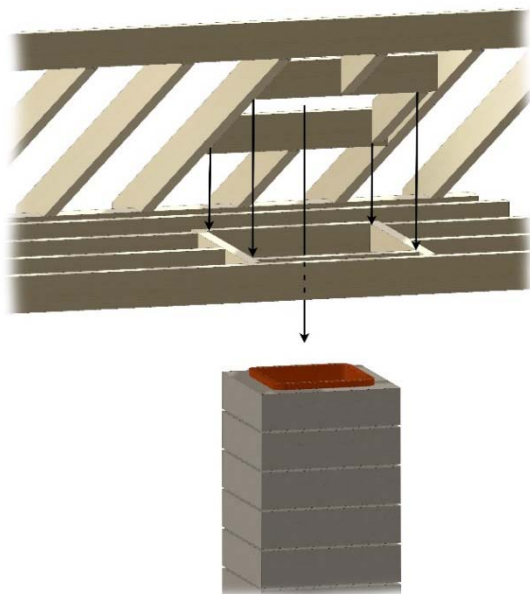
Figura 23. Penetración en el techo
