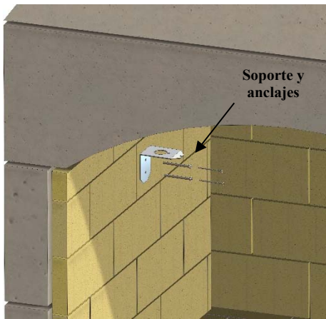
Figura 27. Instalar el soporte y los anclajes
