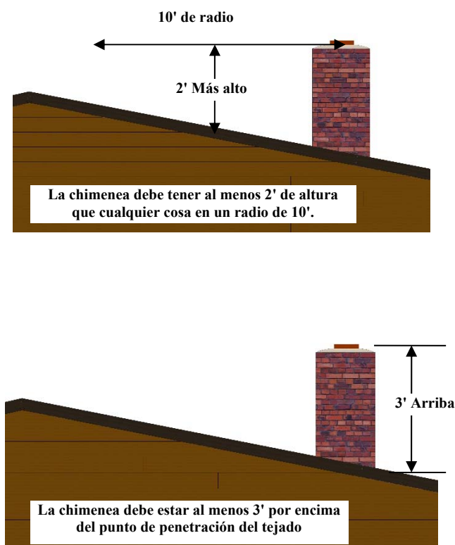
Figura 25. Altura de la chimenea
