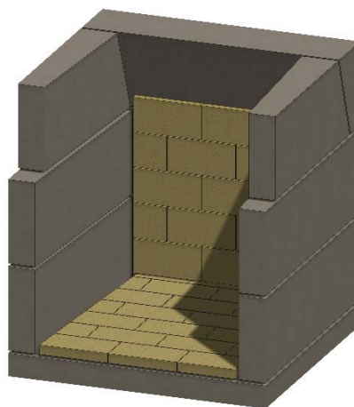
Figura 16. Pared trasera de ladrillo refractario
