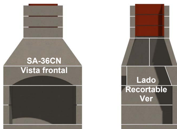
Figura 1. Montaje de la chimenea SA-36CN & Vista en corte
