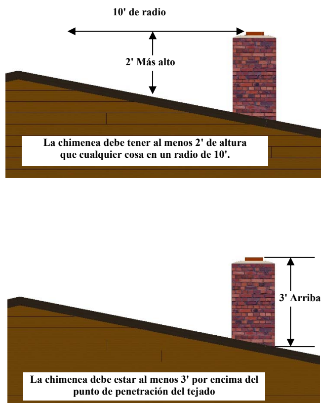
Figura 25. Altura de la chimenea
