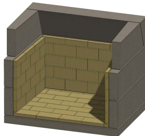
Figura 17. Pared de fuego lateral
