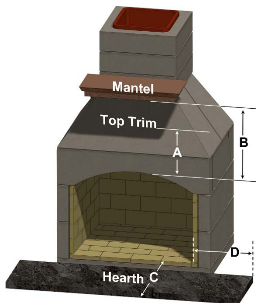
Figura 3. Espacios libres (Utilizar con la tabla 2)
