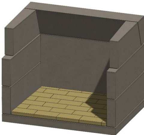
Figura 15. Ladrillo refractario para el suelo
