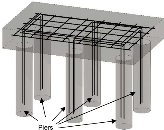
Figura 4. Zapatas con pilares - Vista en corte
