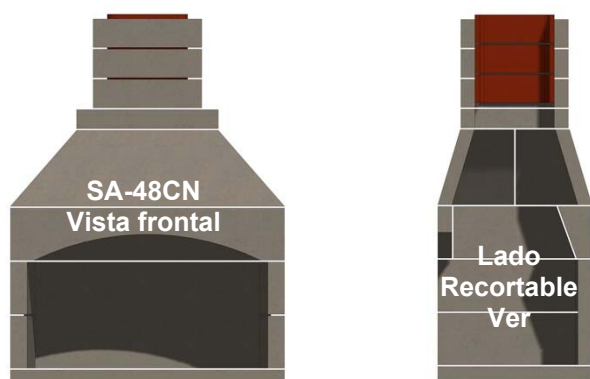
Figura 1. Montaje de la chimenea SA-48CN & Vista en corte
