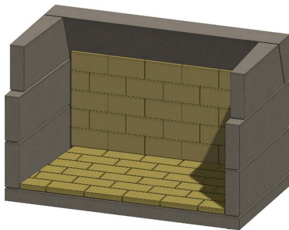
Figura 16. Pared trasera de ladrillo refractario
