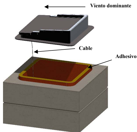
Figura 27. Instalación de la compuerta de montaje superior
