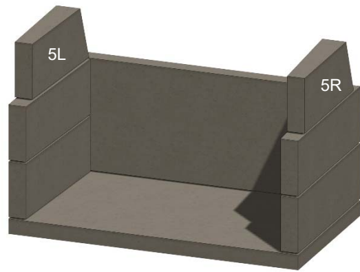
Figura 13. Paredes laterales superiores
