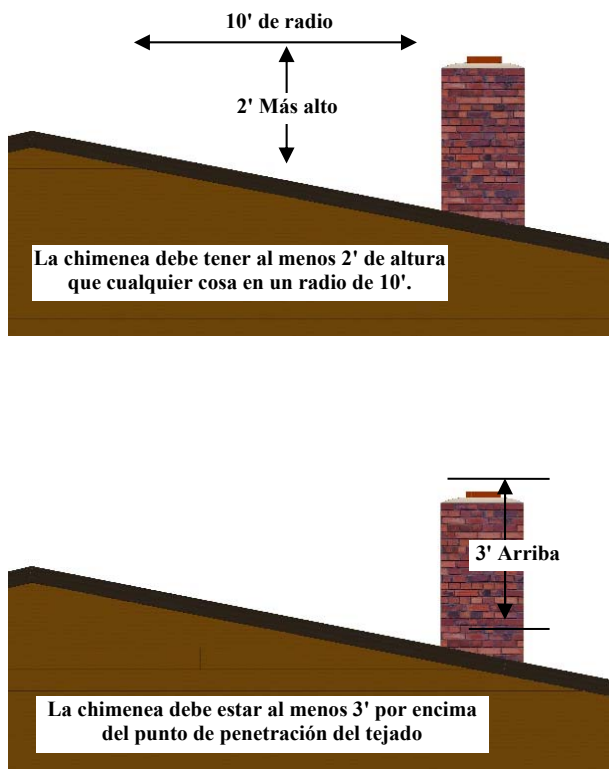
Figura 26. Altura de la chimenea
