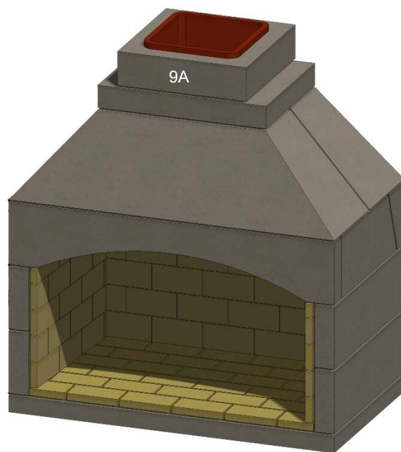
Figura 21. Conducto de la chimenea
