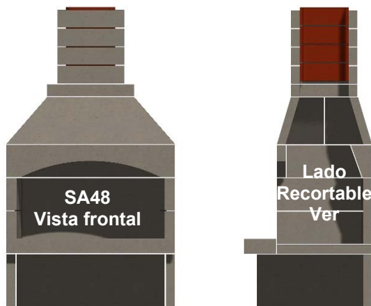
Figura 1. Montaje de la SA48 chimenea & Vista en corte
