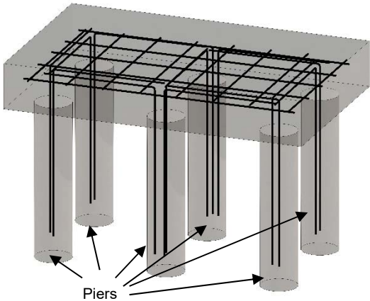
Figura 4. Zapatas con pilares - Vista en corte
