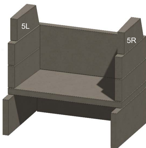
Figura 15. Paredes laterales superiores
