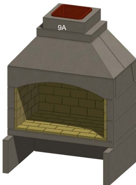
Figura 23. Conducto de la chimenea
