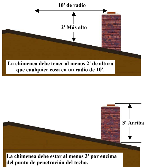
Figura 28. Altura de la chimenea
